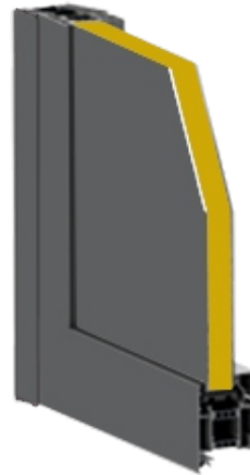
Panel wsadowy - przekrój
